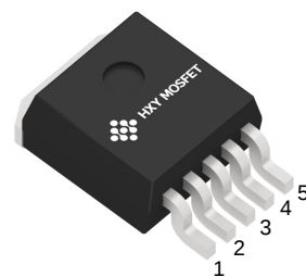
TO-263-5L (DDPAK)
