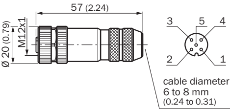
尺寸图 (尺寸单位: mm)
