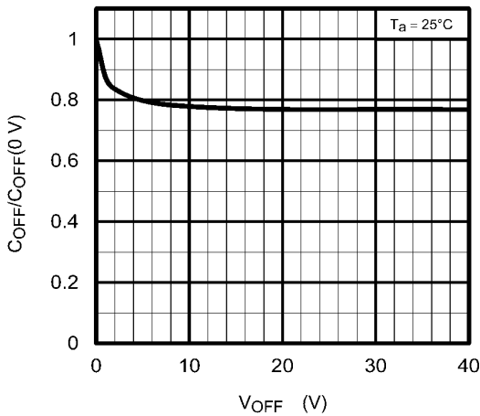
Fig. 12.11 C_{OFF} - V_{OFF}
