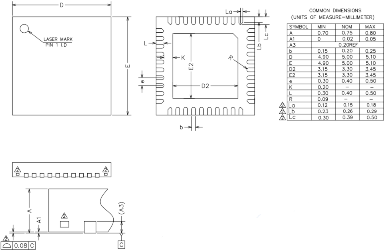
图 10-3 QFN40 封装图
