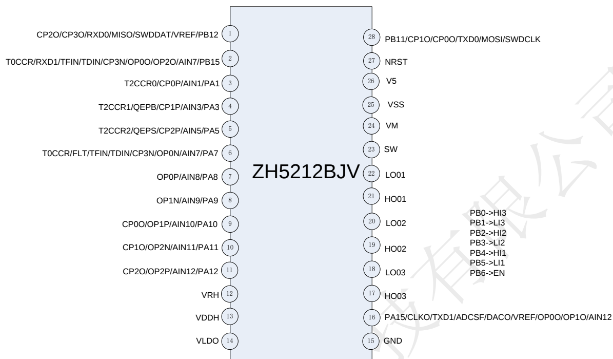
图 3-1-6 ZH5212BJV(ETSSOP28)引脚图
