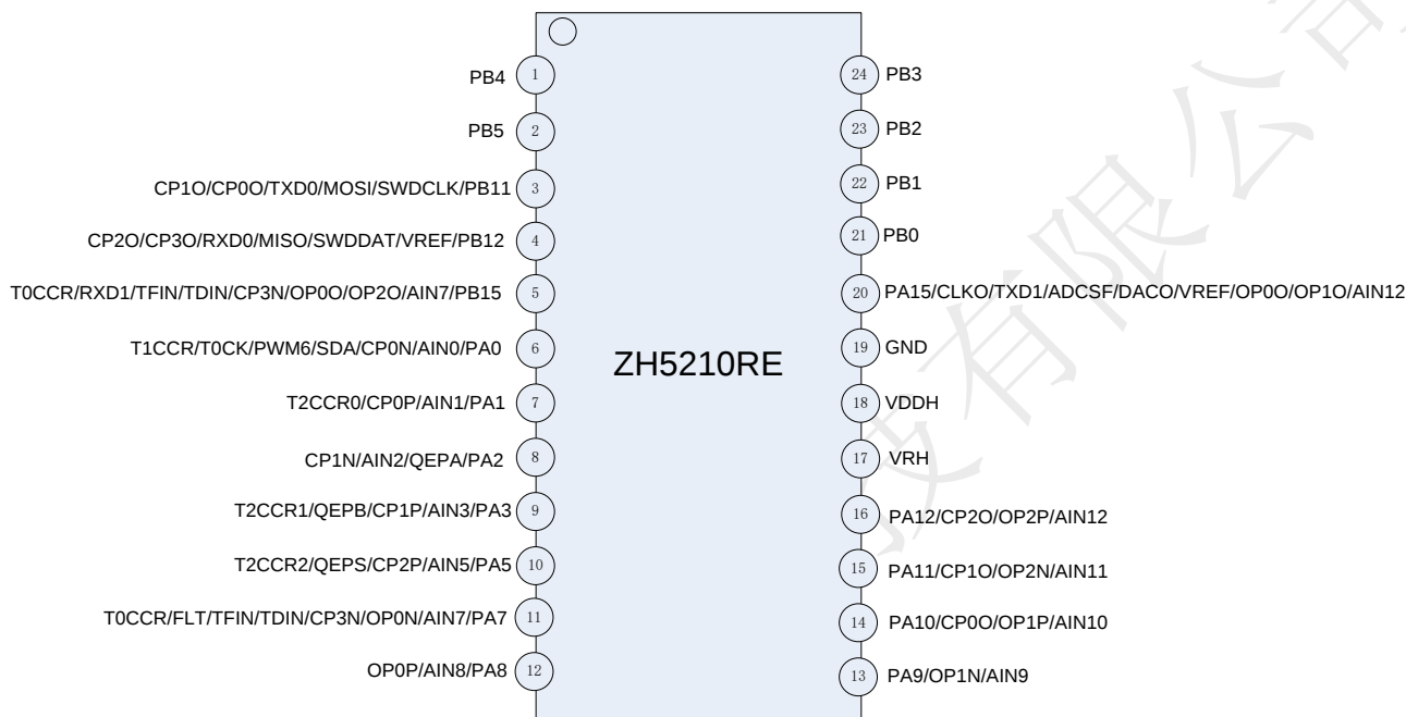
图 3-1-1 ZH5210RE(QSOP24)引脚图
