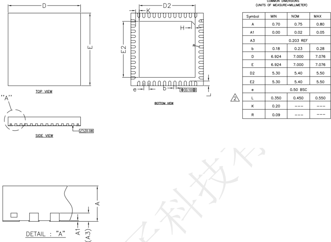
图 10-4 QFN48 封装图
