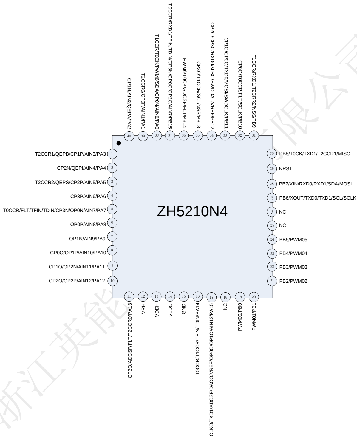
图 3-1-3 ZH5210N4(QFN40)引脚图
