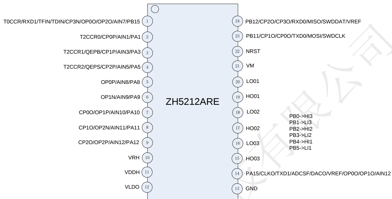
图 3-1-4 ZH5212ARE(QSOP24)引脚图
