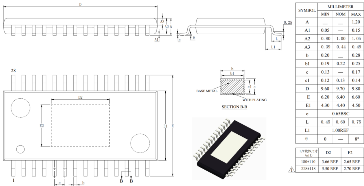
图 10-5 ETSSOP28 封装图
