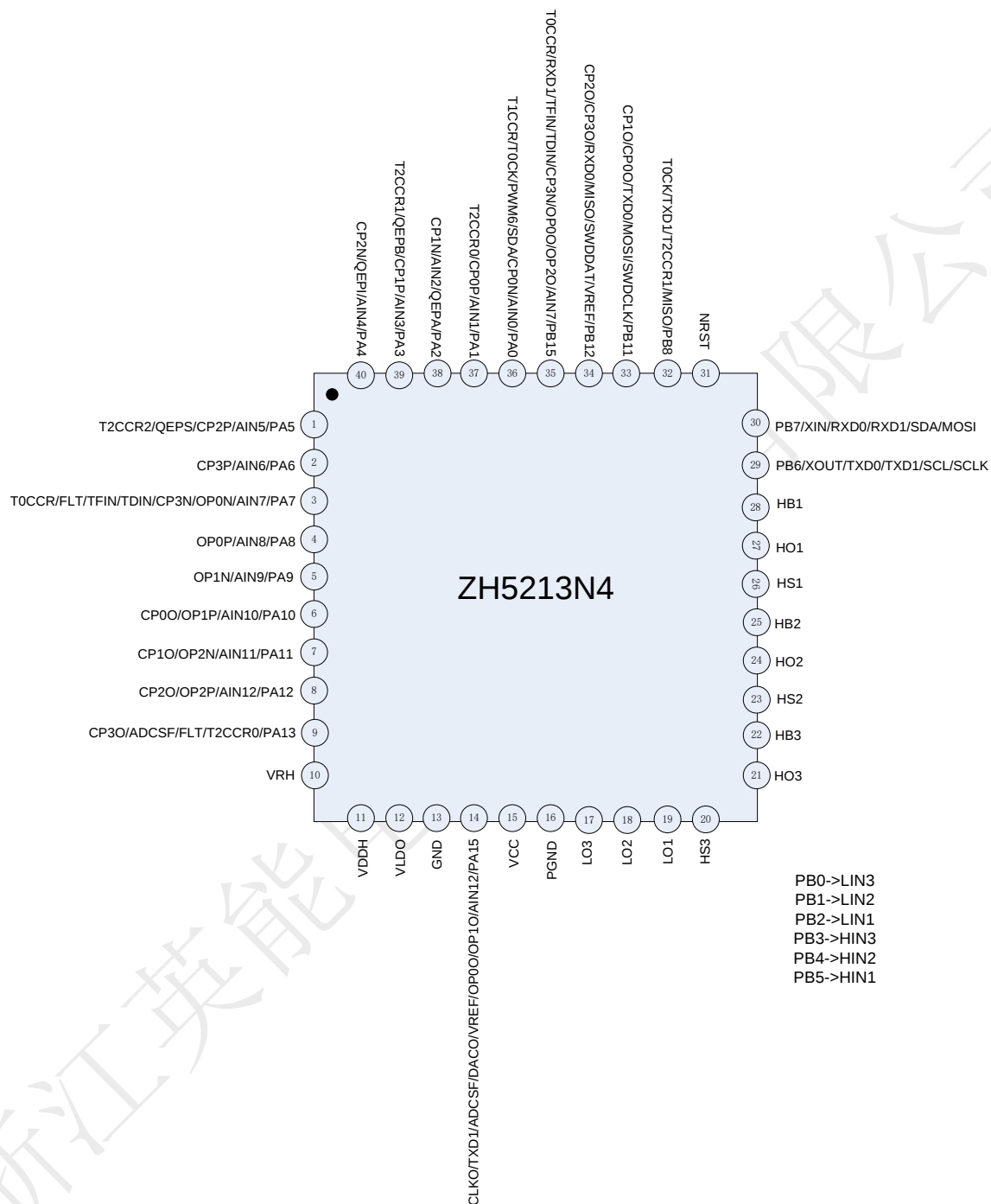
图 3-1-9 ZH5213N4(QFN40)引脚图
