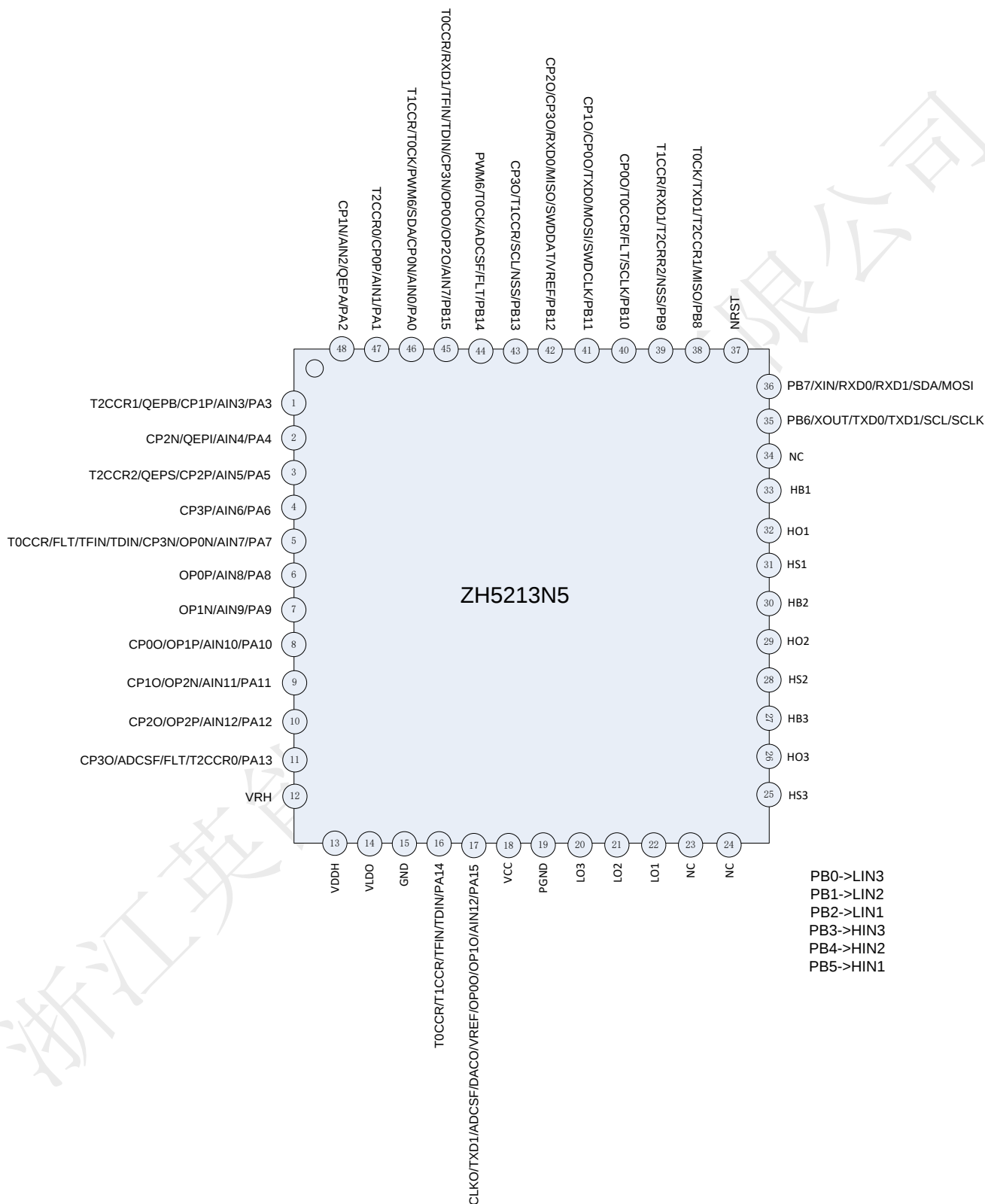
图 3-1-8 ZH5213N5(QFN48)引脚图
