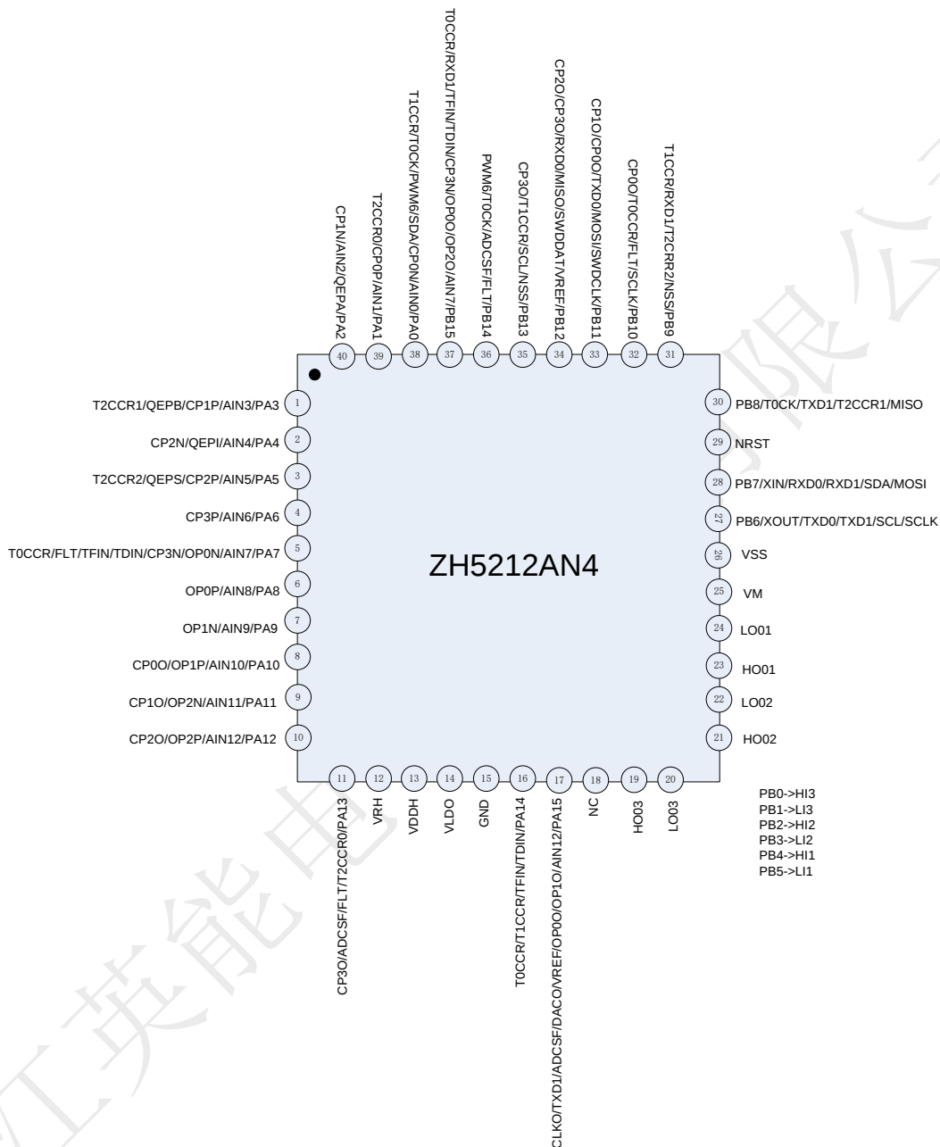
图 3-1-5 ZH5212AN4(QFN40)引脚图
