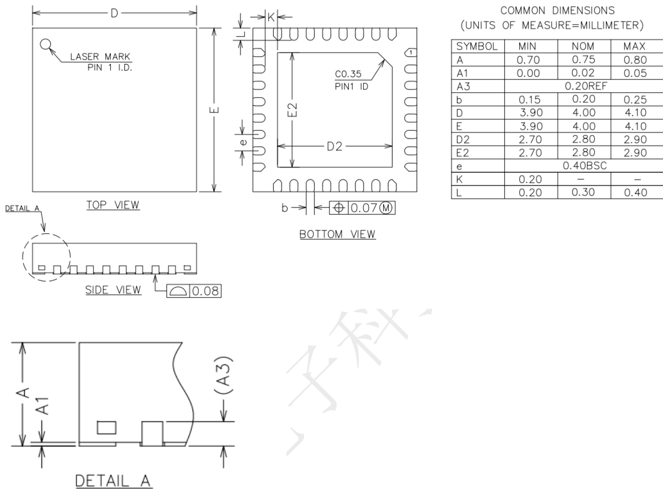
图 10-6 QFN32 封装图
