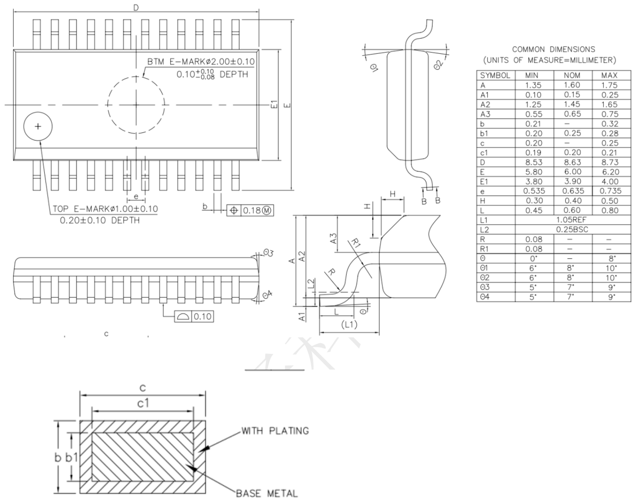
图 10-2 QSOP24 封装图
