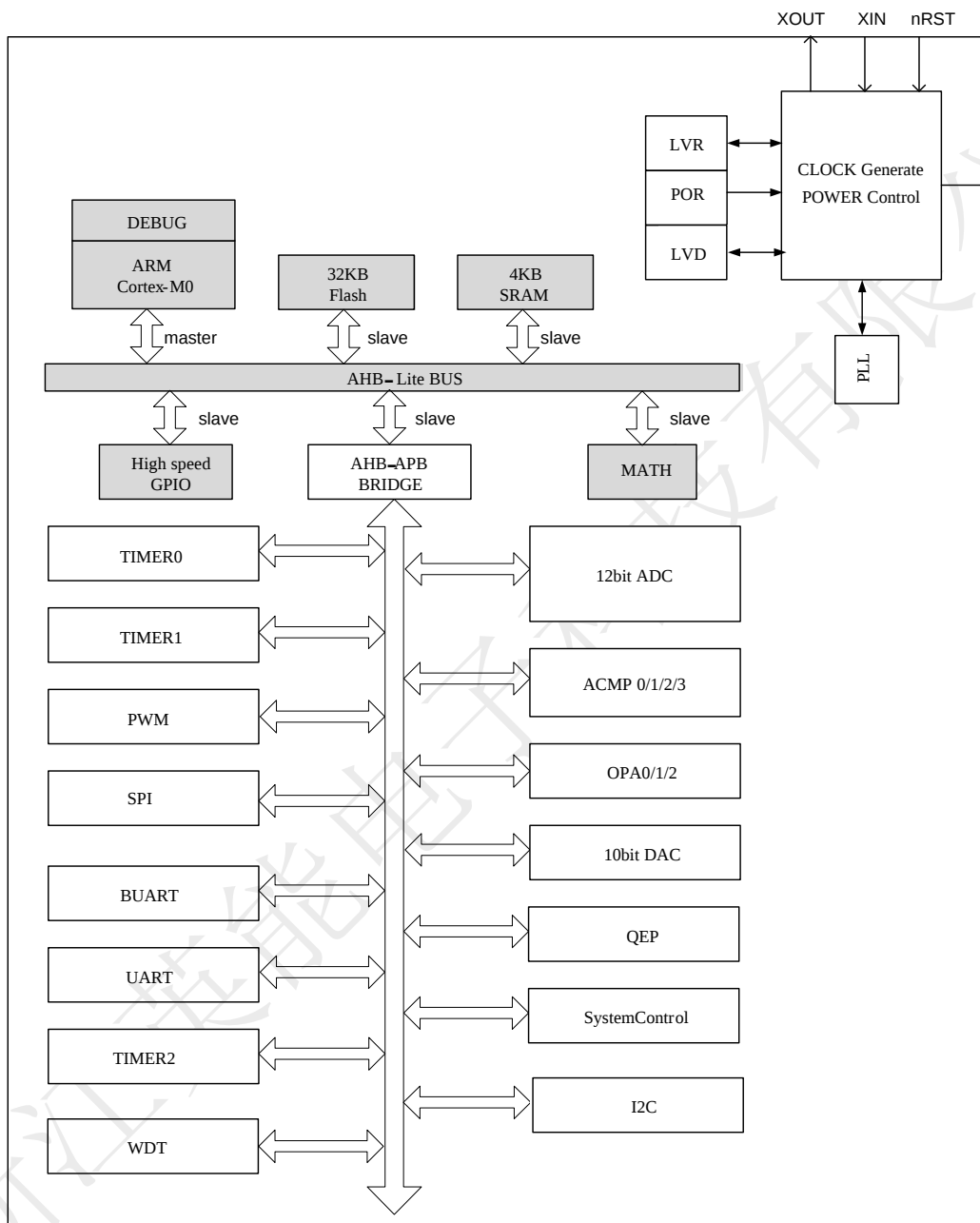
图 2-1 ZH5210 结构框图
