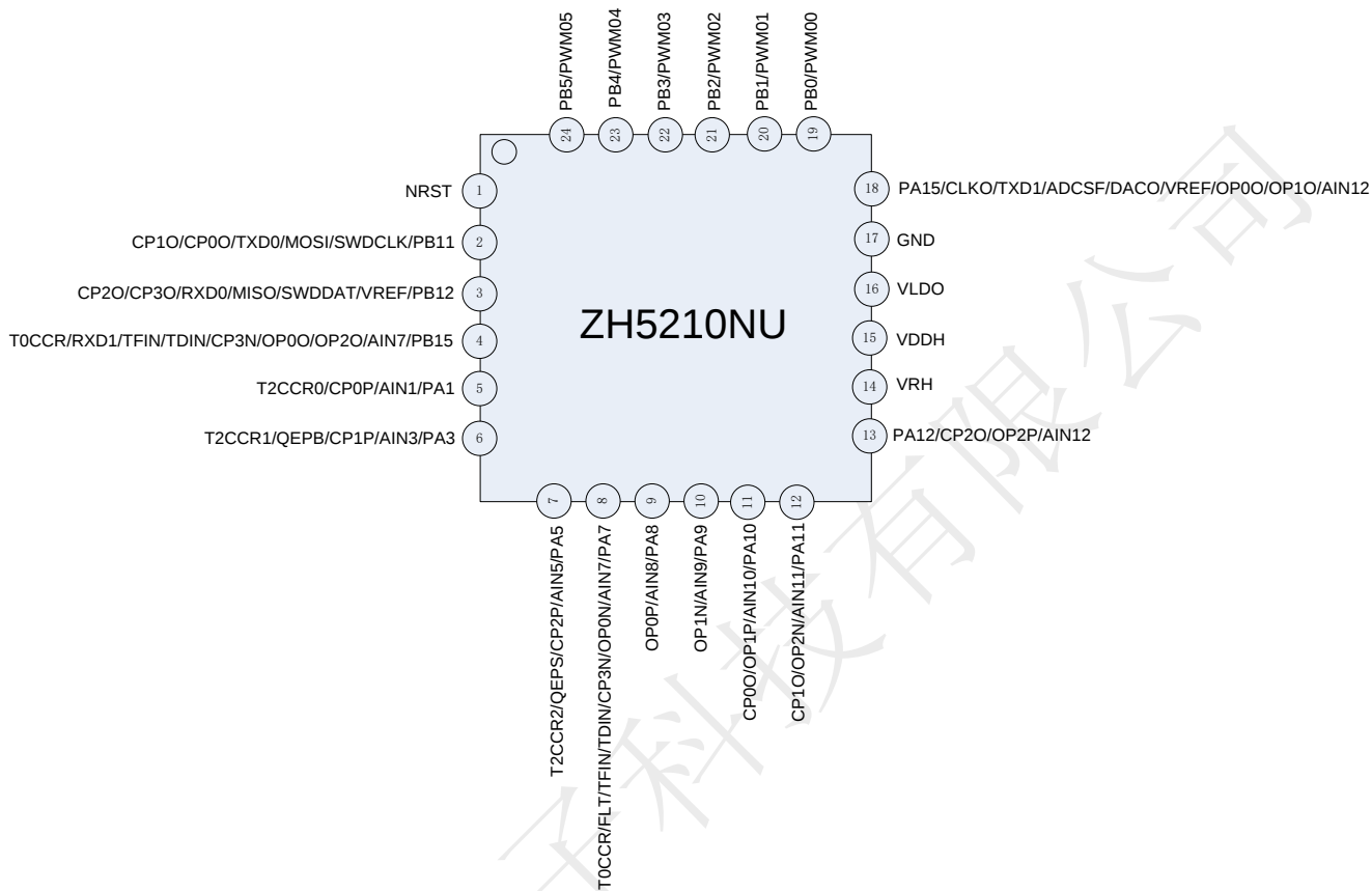
图 3-1-2 ZH5210NU(QFN24)引脚图
