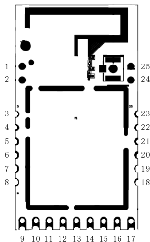
图 2 引脚分布
