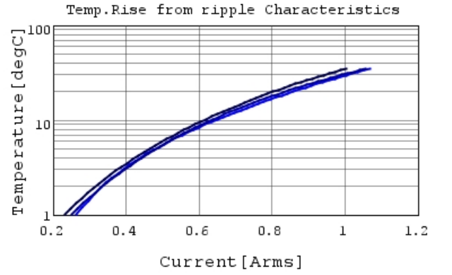
GQM2195G2E2R7BB12 Temp.rise 1GHz 2
