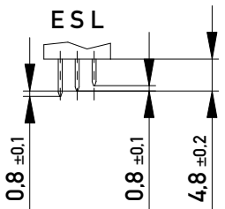
Stecklänge / mating length
