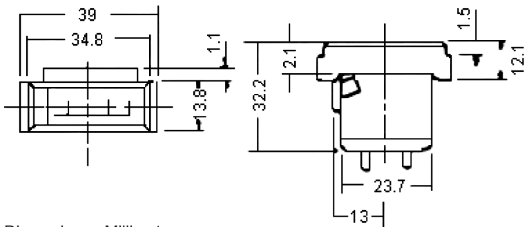
Dimensions : Millimetres
