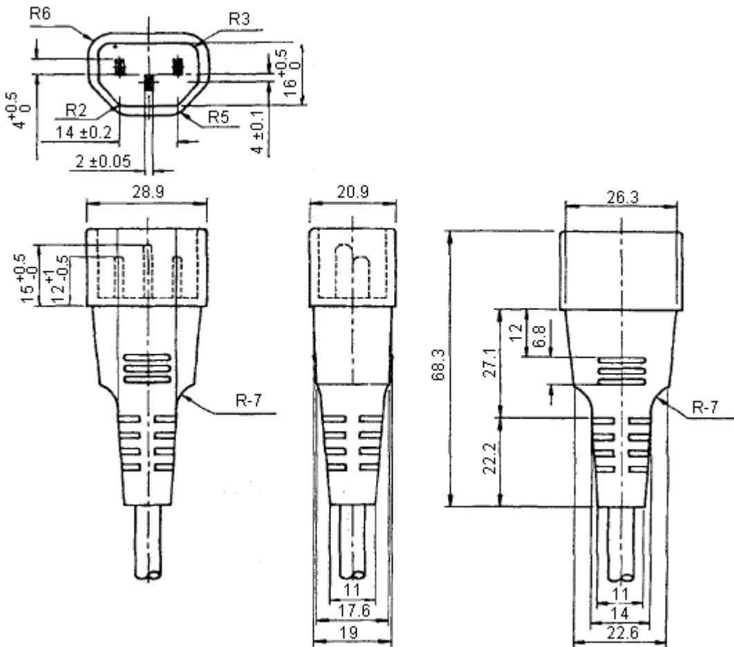
Dimensions : Millimetres
