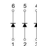
BAS70TW
