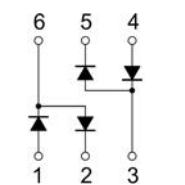
BAS70DW-04
