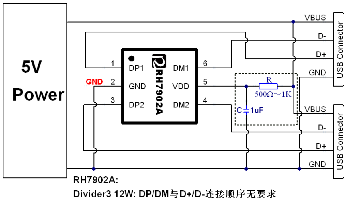
图 3 RH7902A电路示意图
