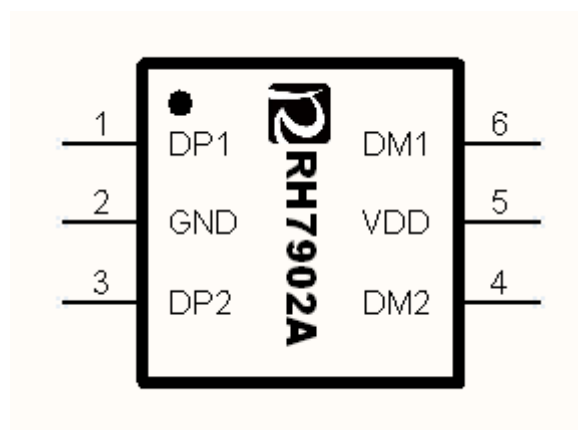
图 1 引脚示意图
