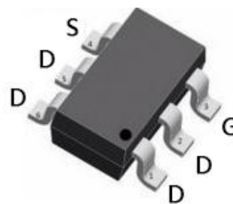
SOT-23-6L
