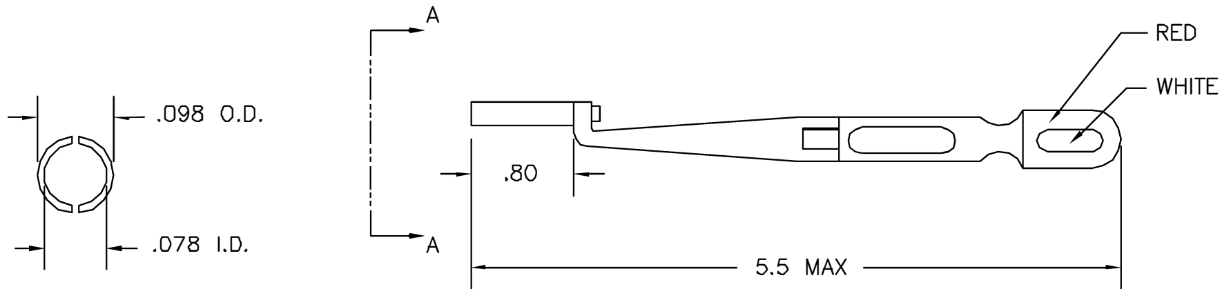
VIEW A-A
