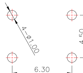
PCB.焊接图
