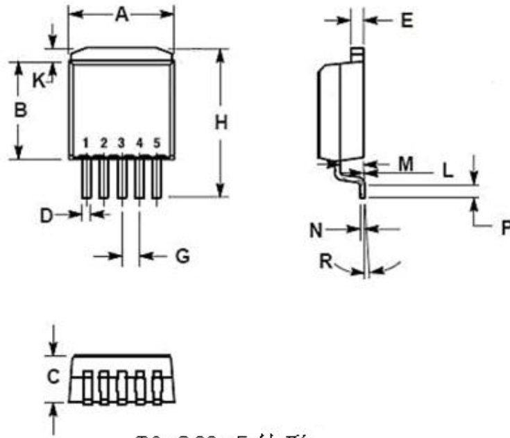
T0-263-5 外形
