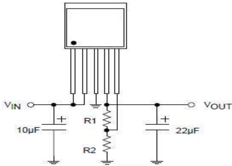
SPX29302典型应用图
