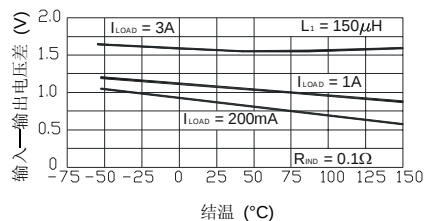
电压降落
