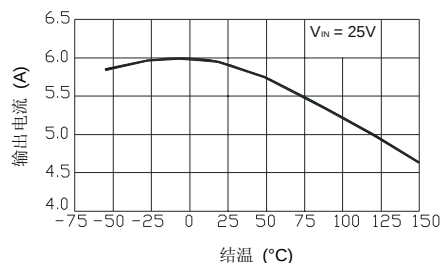
电流极限值
