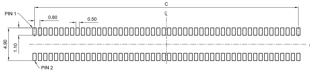
钢网布局
