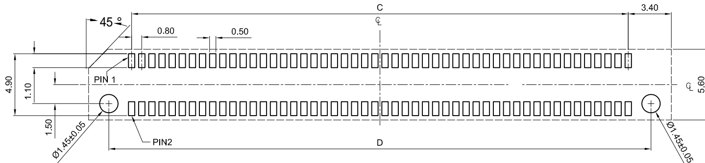
建议印制板引脚排布
