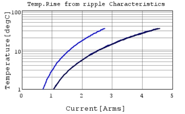
GRM21BR71A225KA01 Temp.rise — 100kHz —
