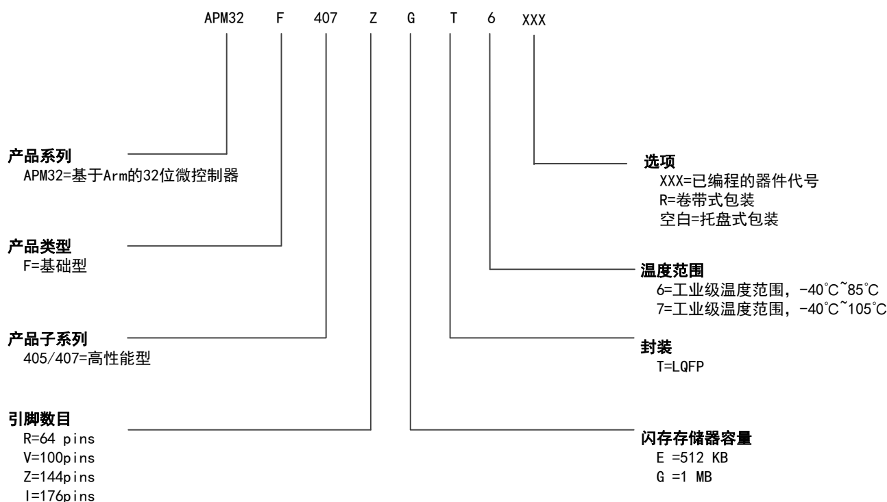
图 31 APM32F405xG 407xExG 系列订货信息图
