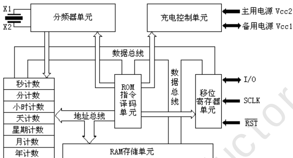
图 1 JSM1302Z内部框图
