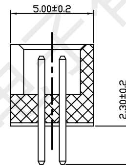
A-A SECTION
