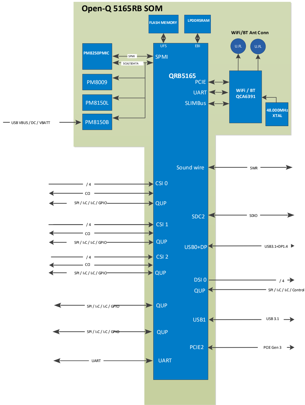
Figure 1. Open-Q 5165RB SOM Block Diagram
