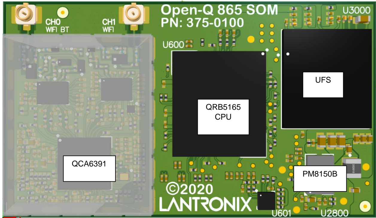
Figure 2. Open-Q 5165RB SOM Top View
