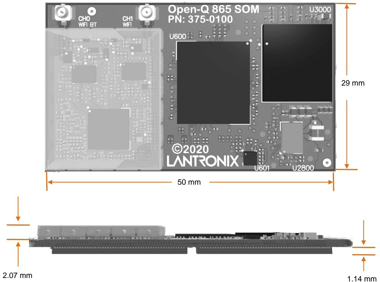
Figure 6. SOM Mechanical Outline
