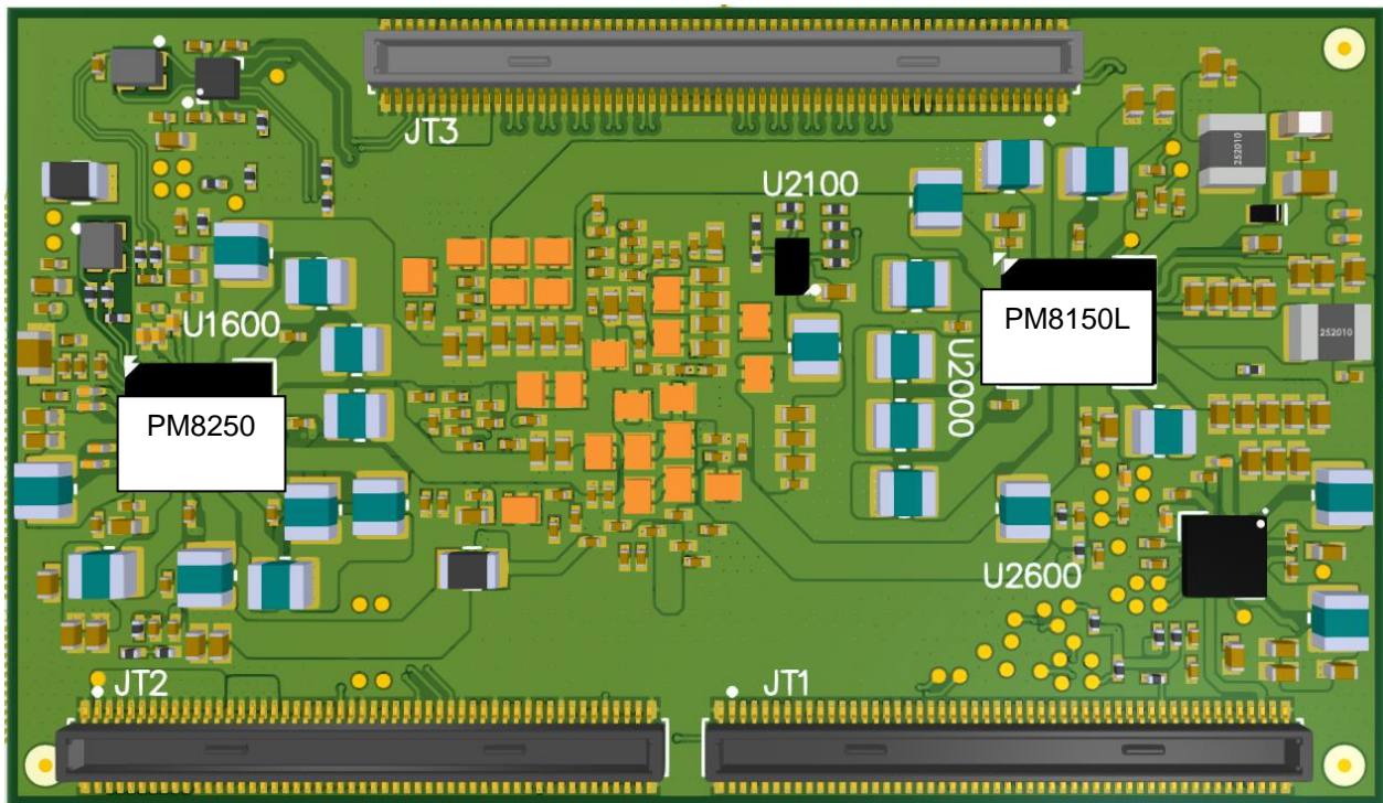
Figure 3. Open-Q 5165RB SOM Bottom View
