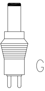
Klinkenstecker/ jackplug 3,5x15mm Art.Nr.:10950037
