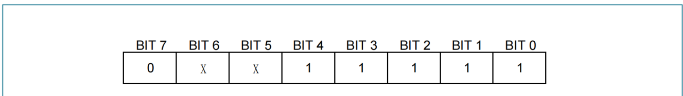
图 8. 配置寄存器
