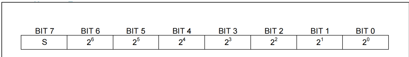
图 3. TH 和 TL 寄存器格式
