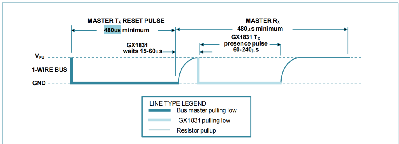
图 13. 初始化序列
