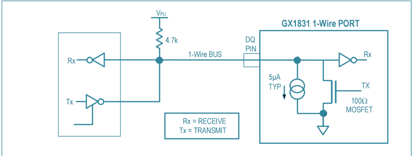
图 10. 硬件结构图
