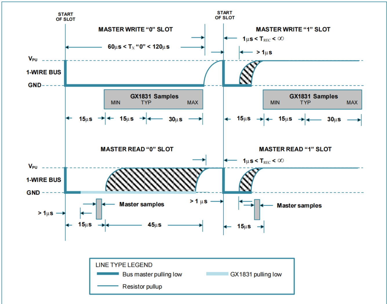
图 14. 读/写时隙时序图
