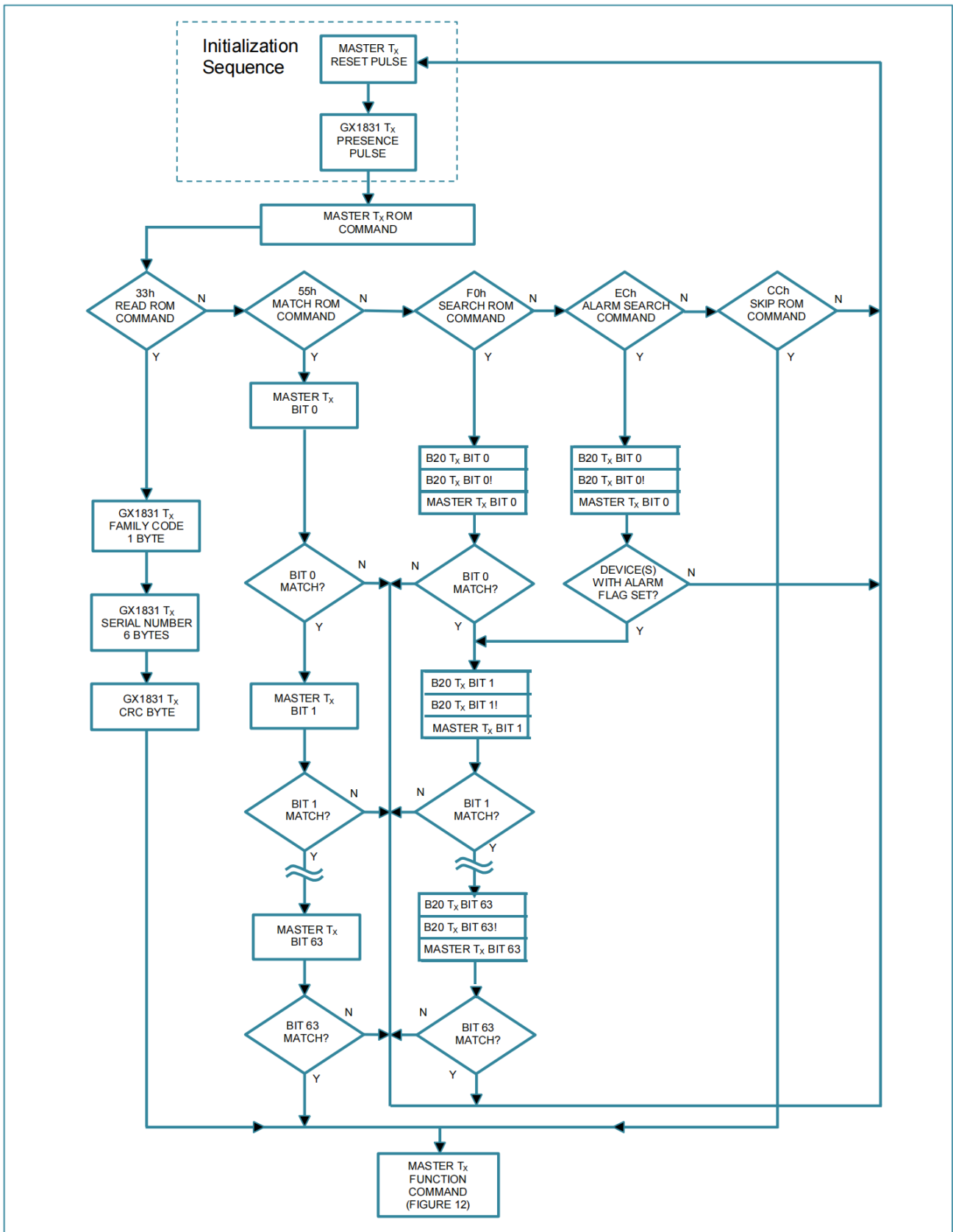
图 11. ROM 指令流程图
