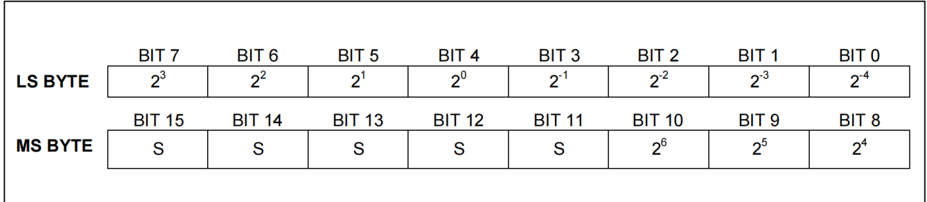
图 2. 温度寄存器格式
