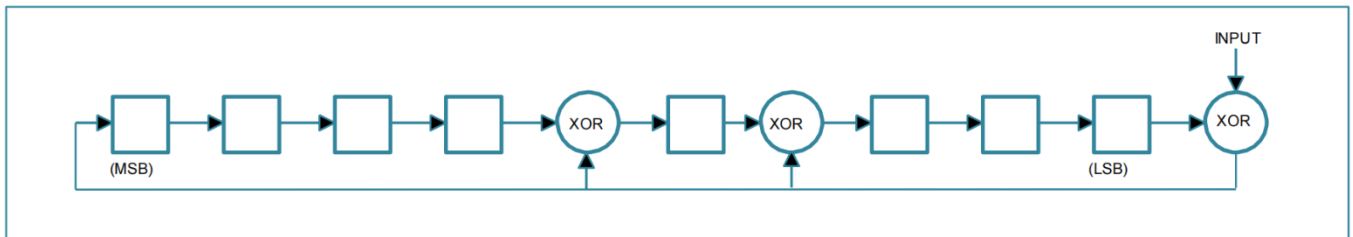
图 9. CRC 产生器
