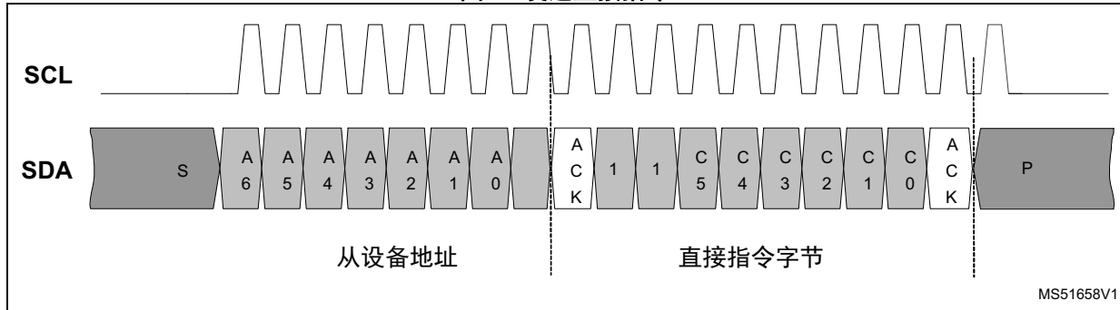
图22. 发送直接指令
