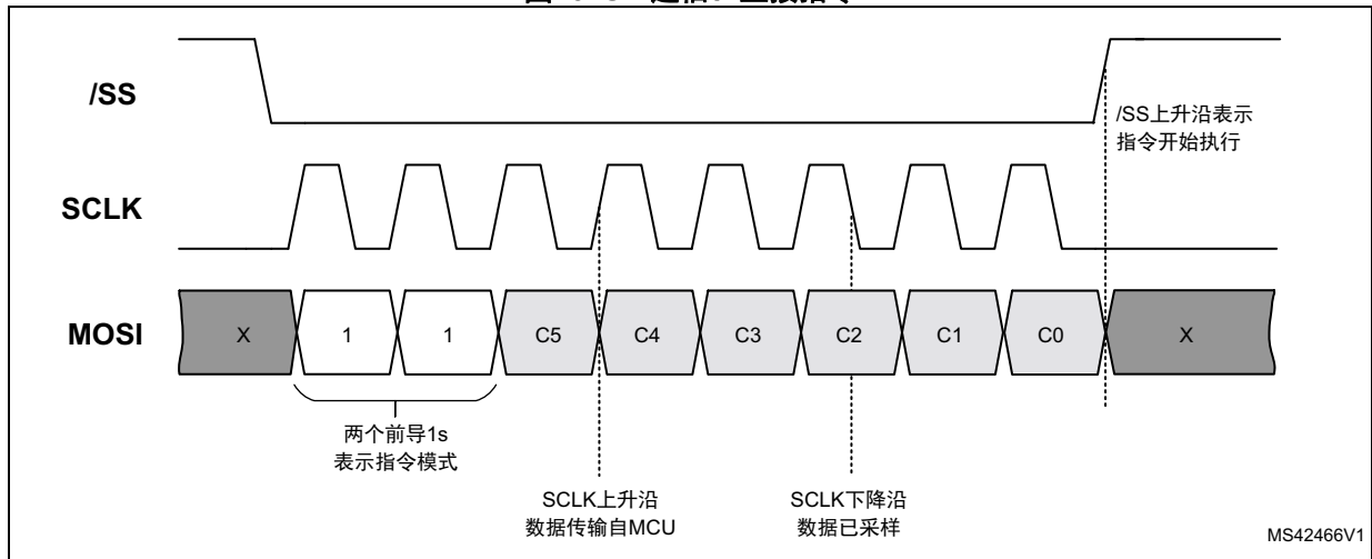
图15. SPI通信：直接指令
