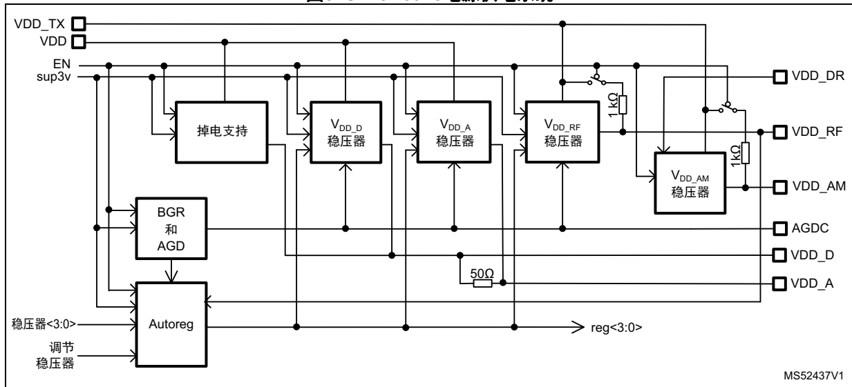
图8. ST25R3918电源供电系统
