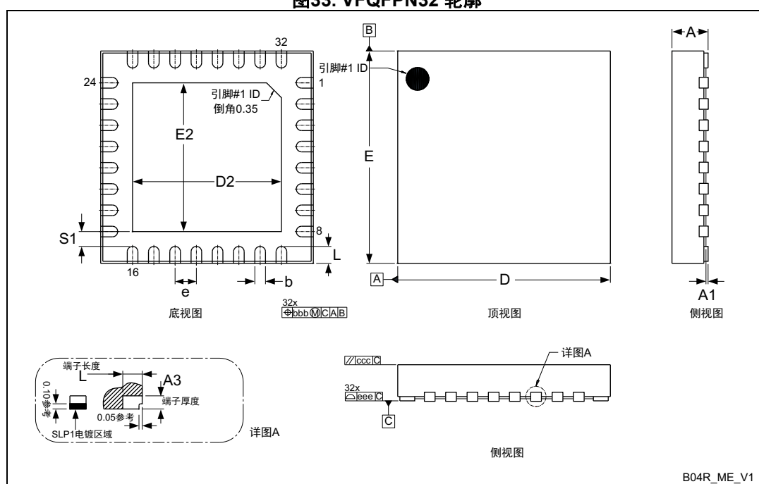
图33. VFQFPN32 轮廓
