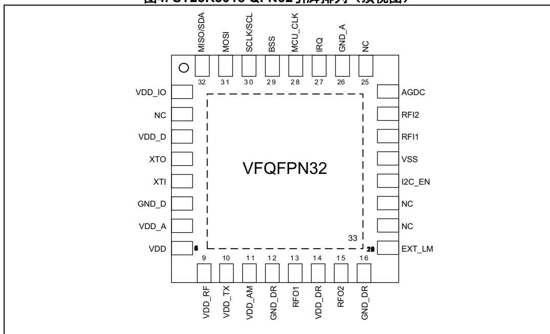
图4. ST25R3918 QFN32引脚排列 (顶视图)
