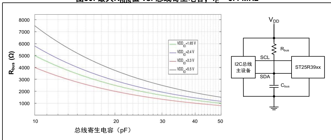
图30. 最大 R_{bus} 值 vs. 总线寄生电容, f_c = 3.4 MHz
