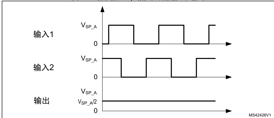
图6. 90^\circ 相移情况下，相位检测器输入和输出
