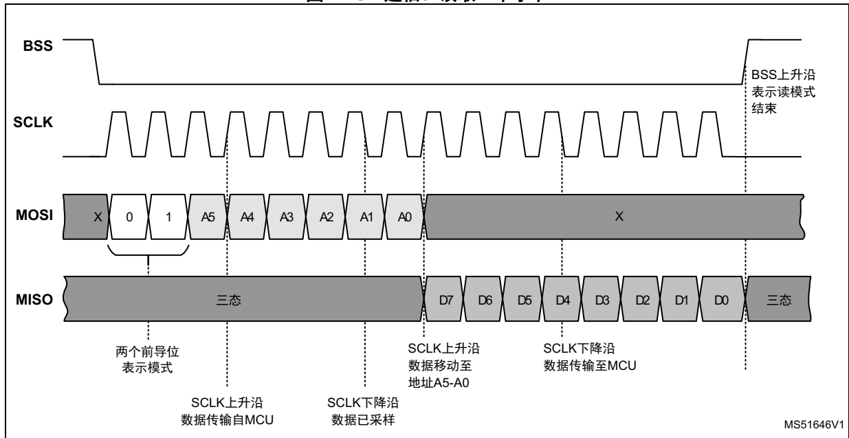
图12. SPI通信：读取一个字
