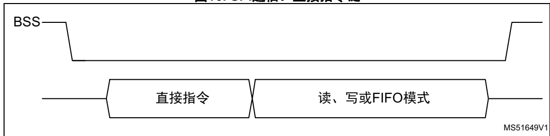
图16. SPI通信：直接指令链
