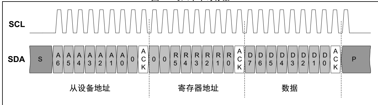
图17. 写入单个寄存器
