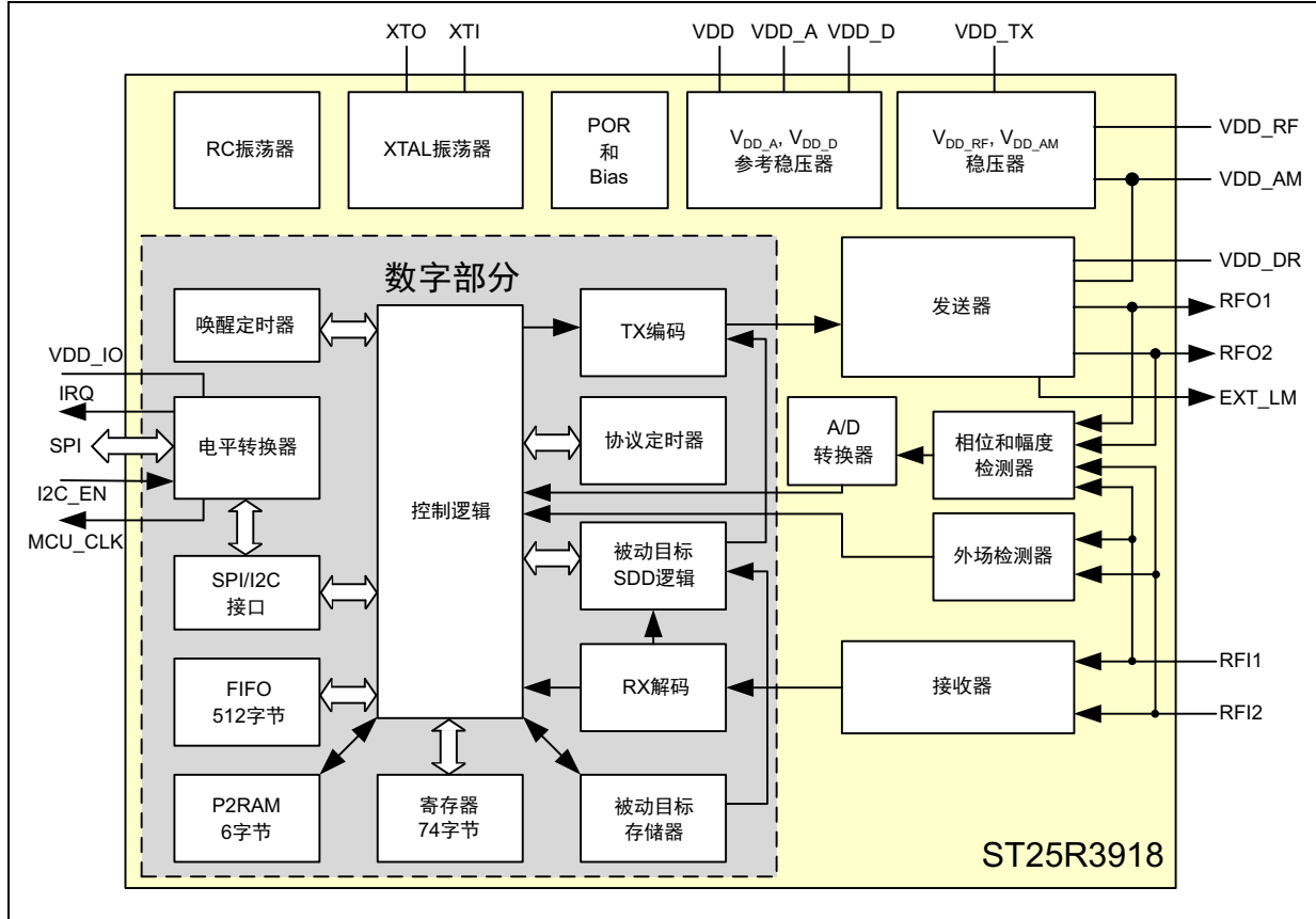
图3. ST25R3918框图
