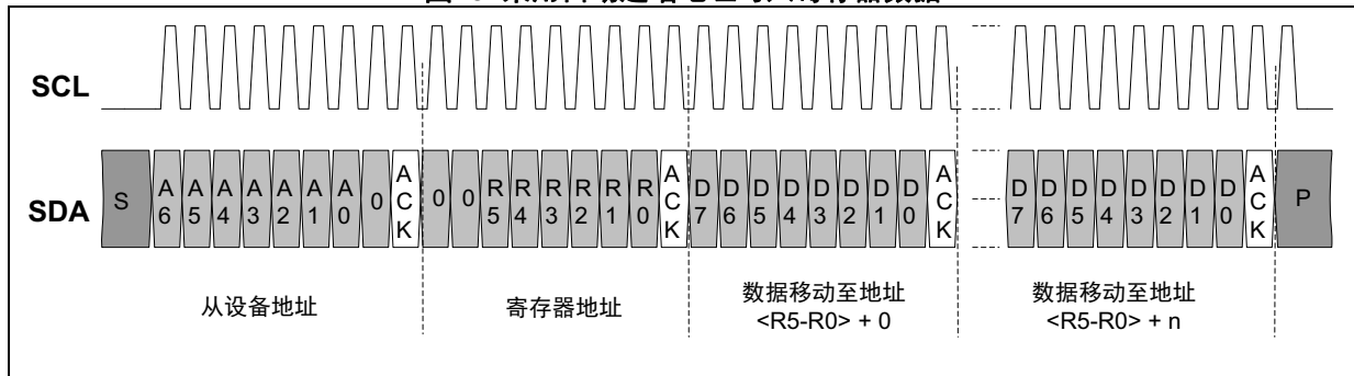
图18. 采用自动递增地址写入寄存器数据
