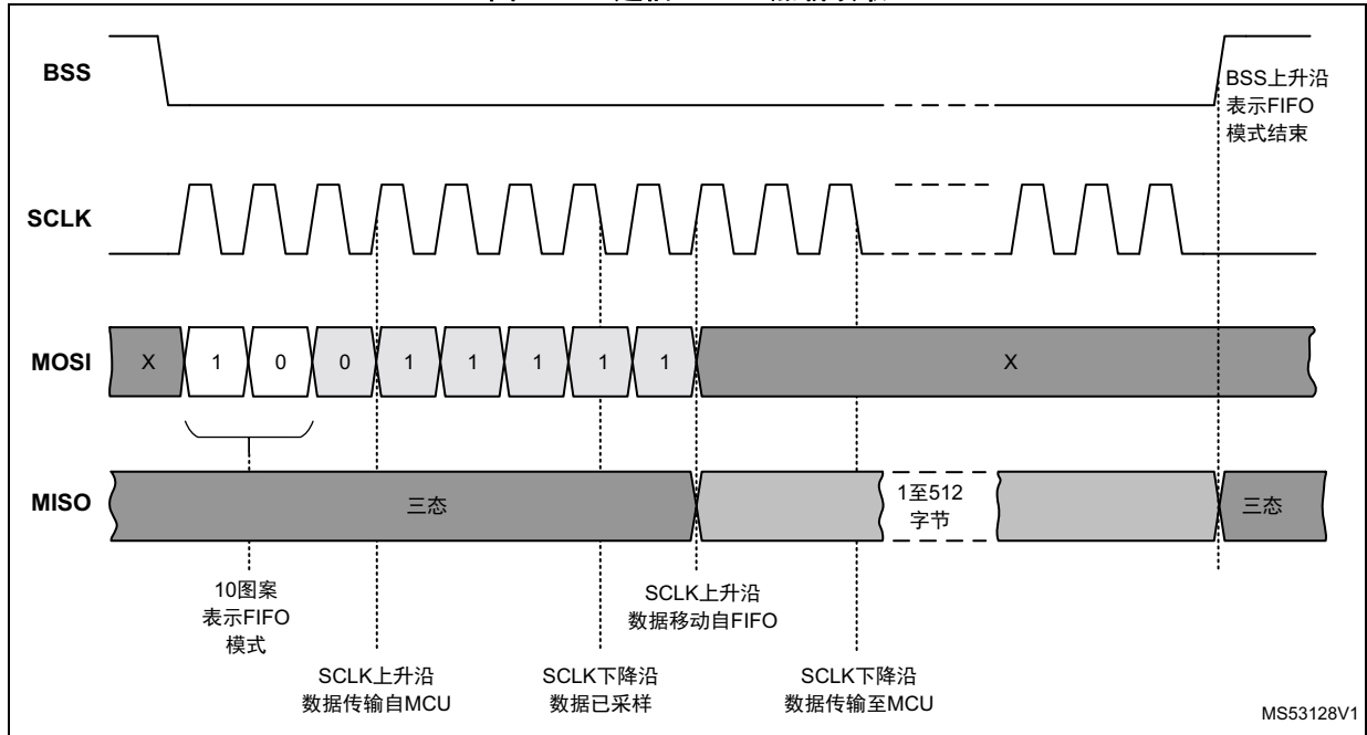
图14. SPI通信：FIFO加载读取
