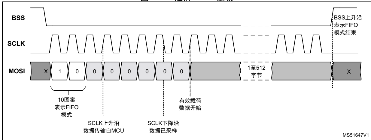
图13. SPI通信：FIFO加载
