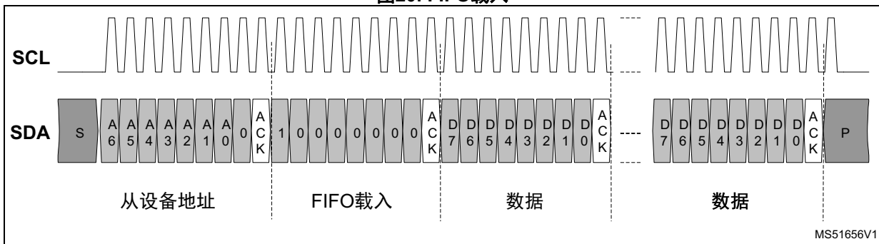
图20. FIFO载入
