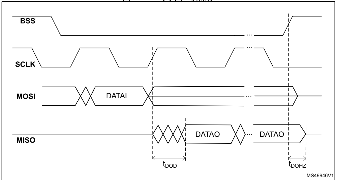
图28. SPI时序图 - 读操作
