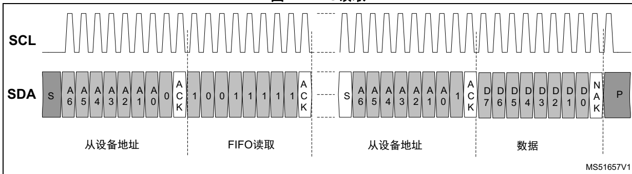
图21. FIFO读取
