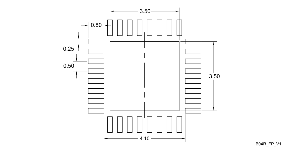
图34. VFQFPN32 建议封装图
