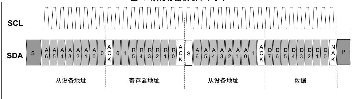
图19. 从寄存器读取单个字节
