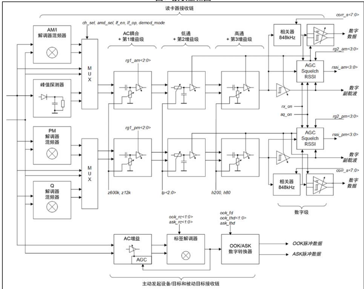
图5. 接收器框图
