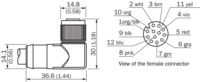
尺寸图 (尺寸单位: mm)
