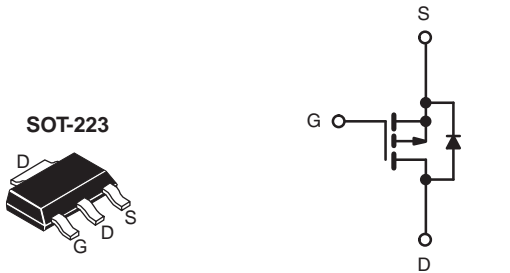
P-Channel MOSFET
