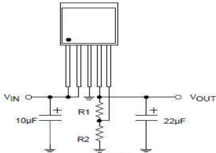
MIC29302WU 典型应用图
