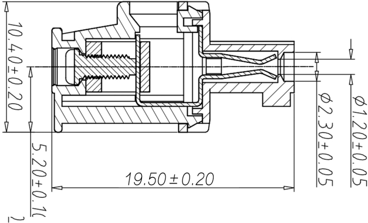
剖面 A-A
