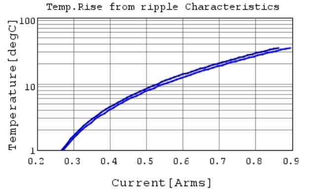
GJM1555C1H2R0BB01 Temp.rise — 2GHz — 3
