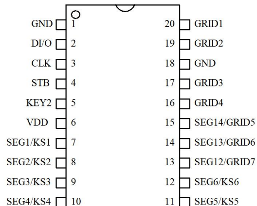
TM1620B SOP-20
