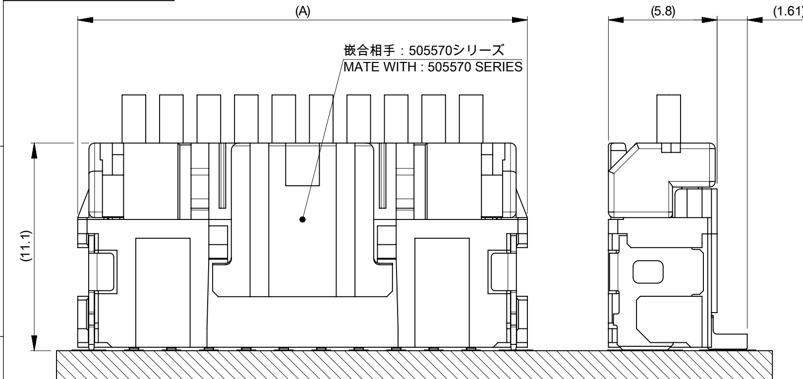
嵌合状態図 MATED CONNECTOR
