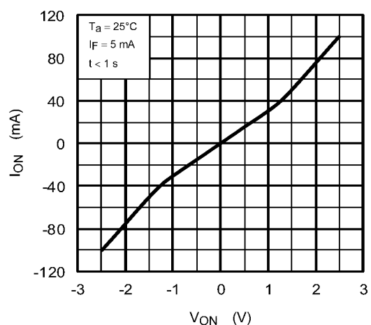
Fig. 14.4 I_{ON} - V_{ON}
