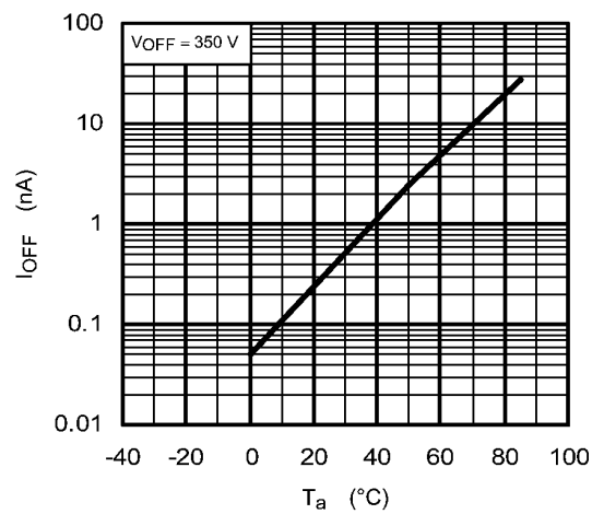
Fig. 14.9 I_{OFF} - T_a
