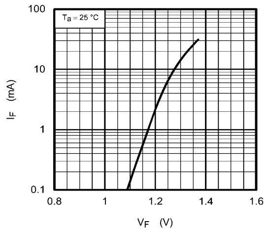
Fig. 14.3 I_F - V_F
