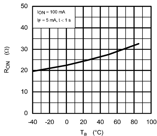
Fig. 14.5 R_{ON} - T_a
