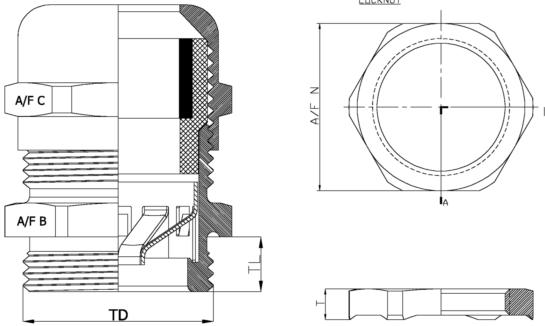
SECTION A-A
