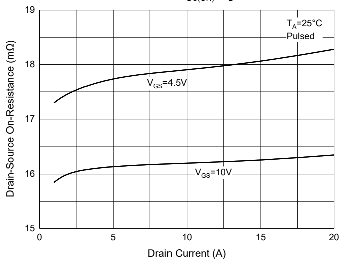
Fig. 5 - R_{DS(ON)} - I_D
