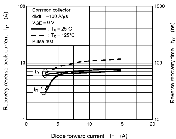
Fig. 8.15 I_{RR} , t_{RR} - I_F
