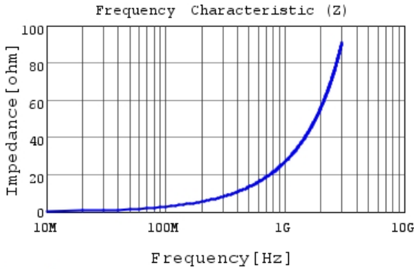
LQP03TN4N3H02 |Z|
