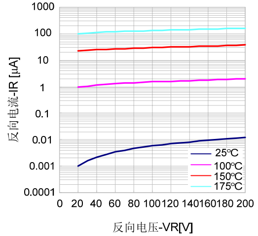
图2: 反向特性
