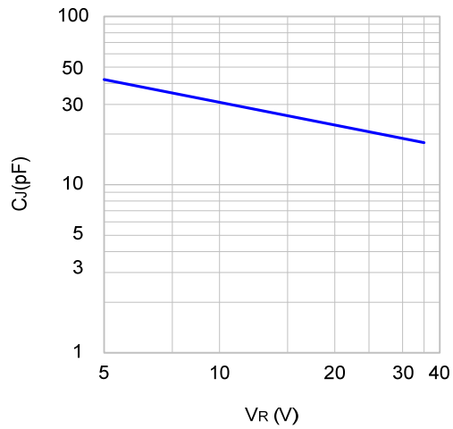
图3: 结电容特性
