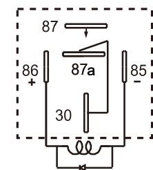
带二极管型 (D1)
