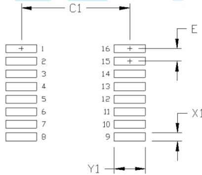
图 25. 16 引脚 SSOIC 封装 [16-Lead SSOP] 焊盘图案
