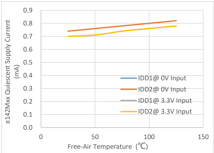
图 13. 3.3V 供电, \pi 142Mxx 静态供电电流 vs. 空气温度
