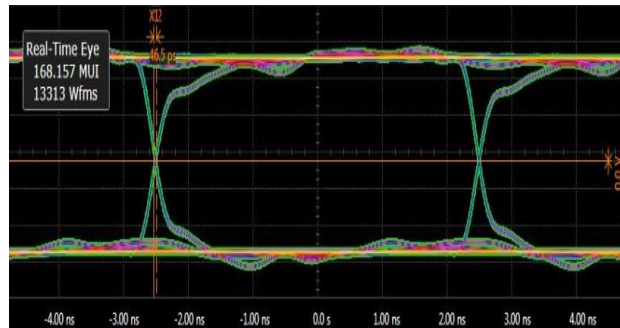
图 18. \pi 14\text{xMxx} 眼图
