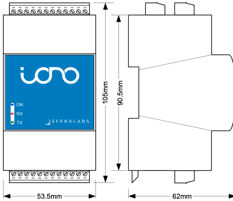
DIMENSIONS
