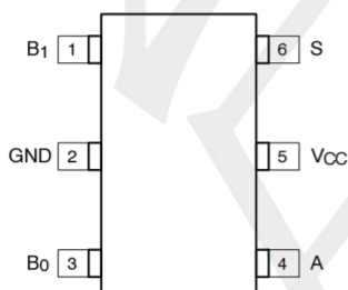
SOT363
