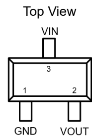
SOT23-3 Package
