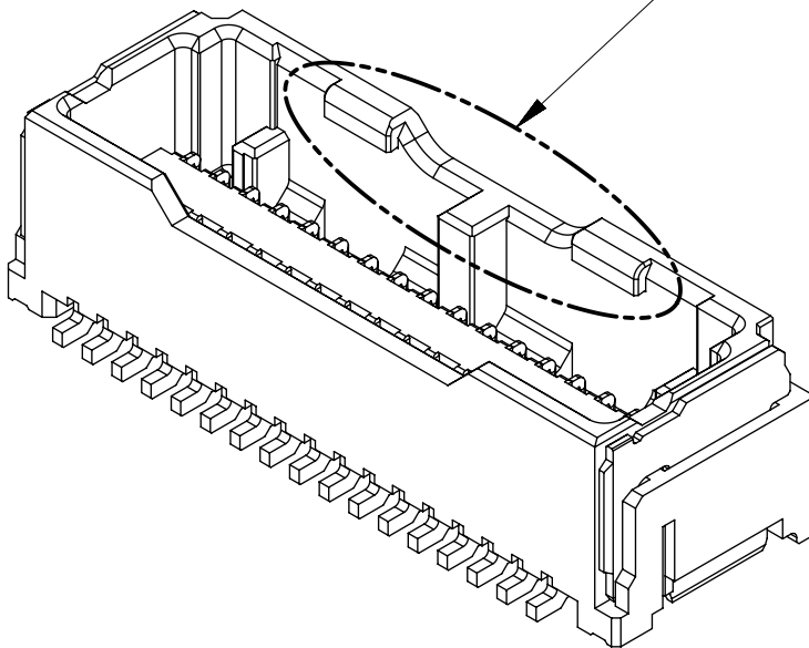
34-42 CKT. 係止形状 LOCK SHAPE OF 34-42 CKT.
