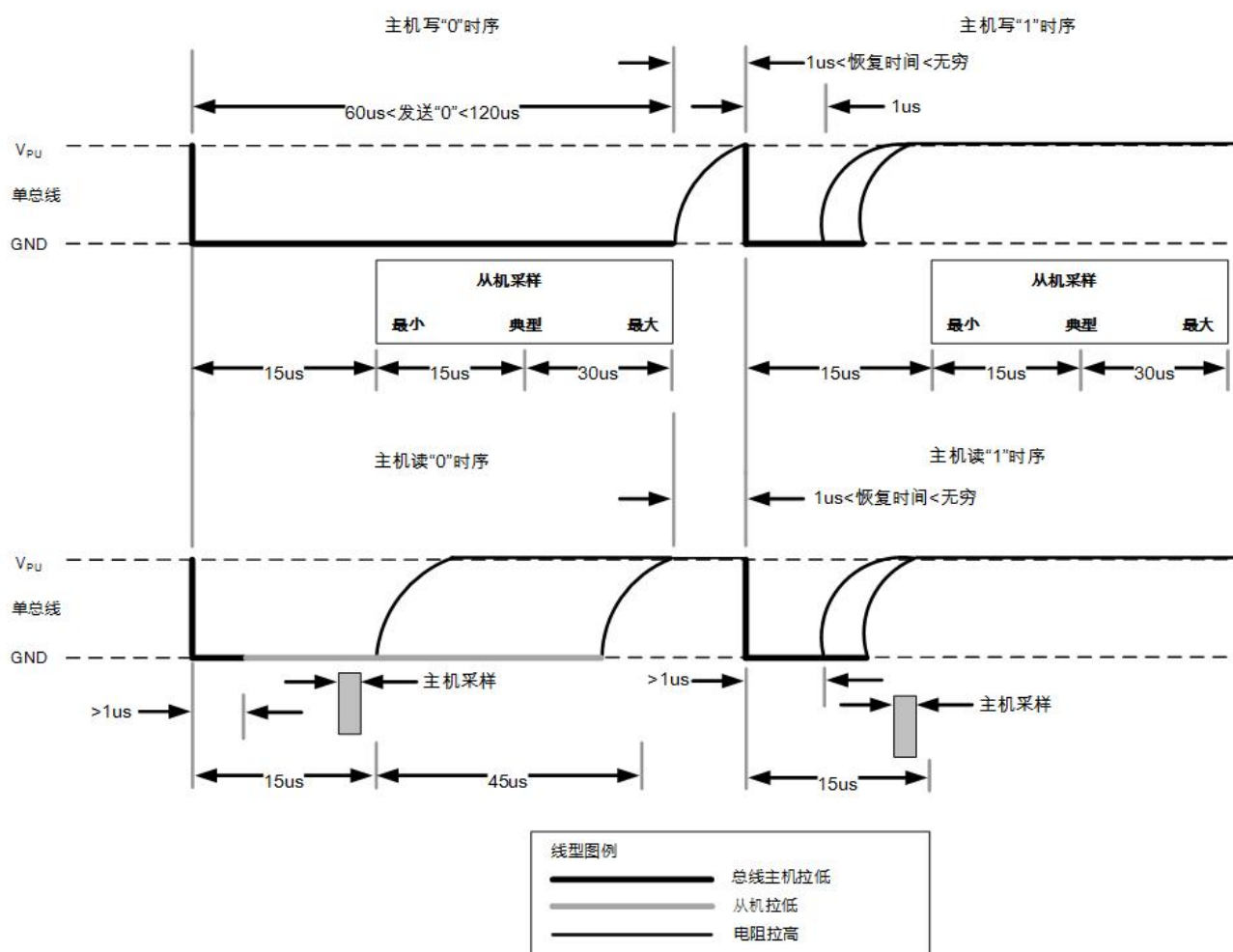
图 12.6-2 读/写时隙时序
