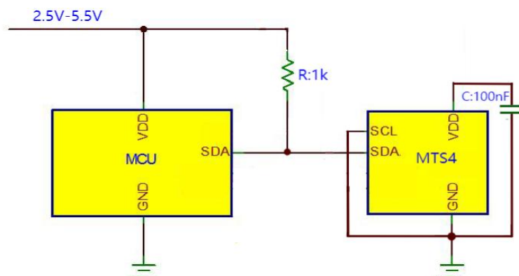
图 9.9-2 寄生模式典型电路图（修改寄存器）
