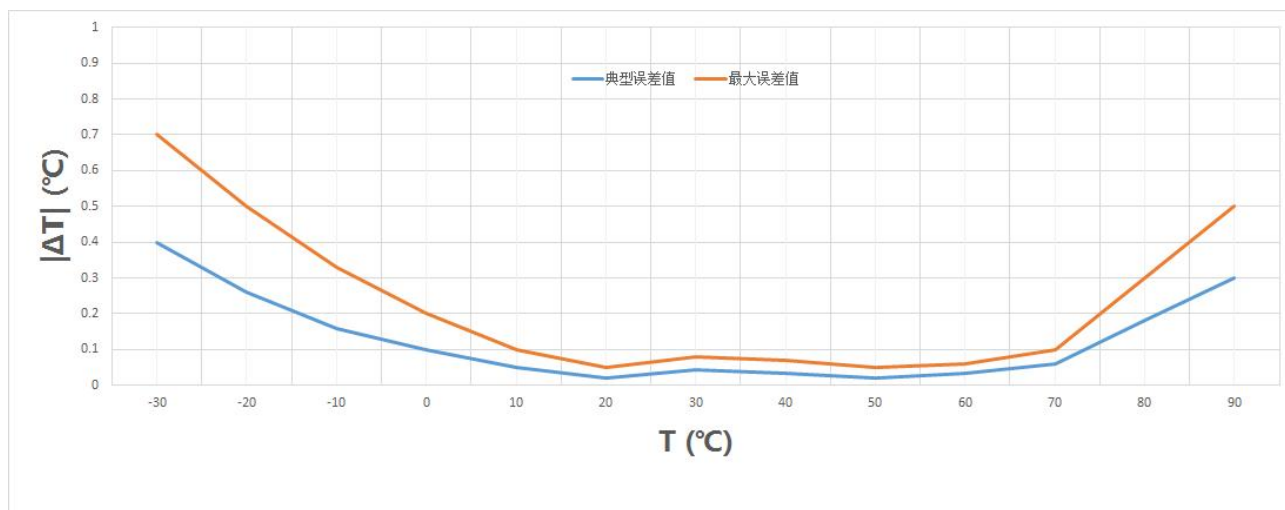
图 7-3 MTS4W 精度误差曲线
