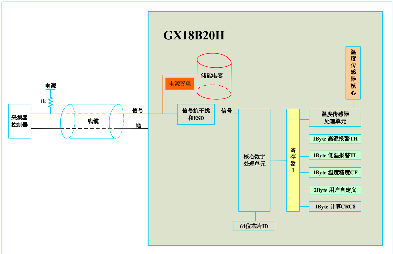
图 1. GX18B20H 结构框图
