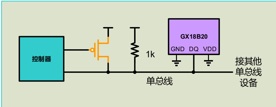
图 4. 在温度转换期间为寄生供电的 GX18B20H 供电
