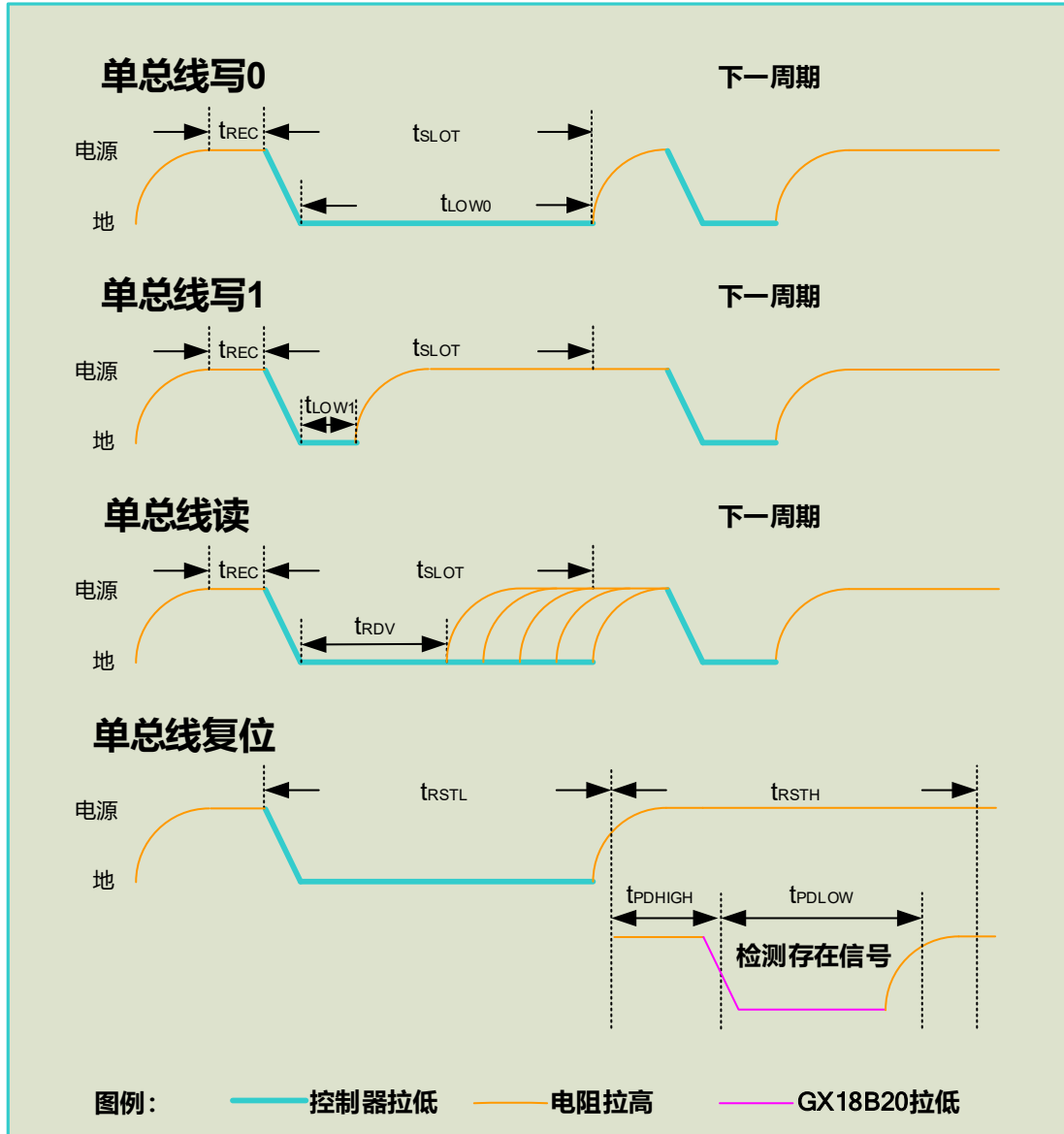
图 17. 时序
