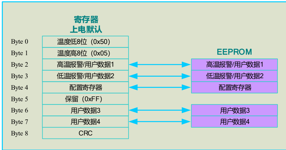
图 7. GX18B20H 存储器图
