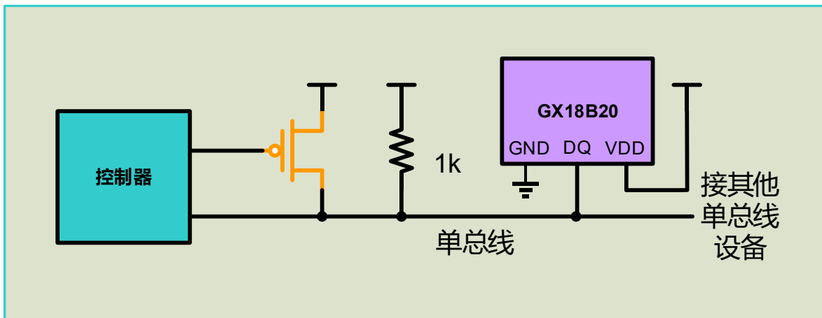
图 5. 使用外部电源为 GX18B20H 供电
