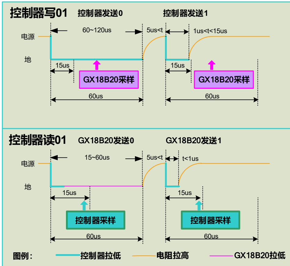
图 14. 读/写时序图
