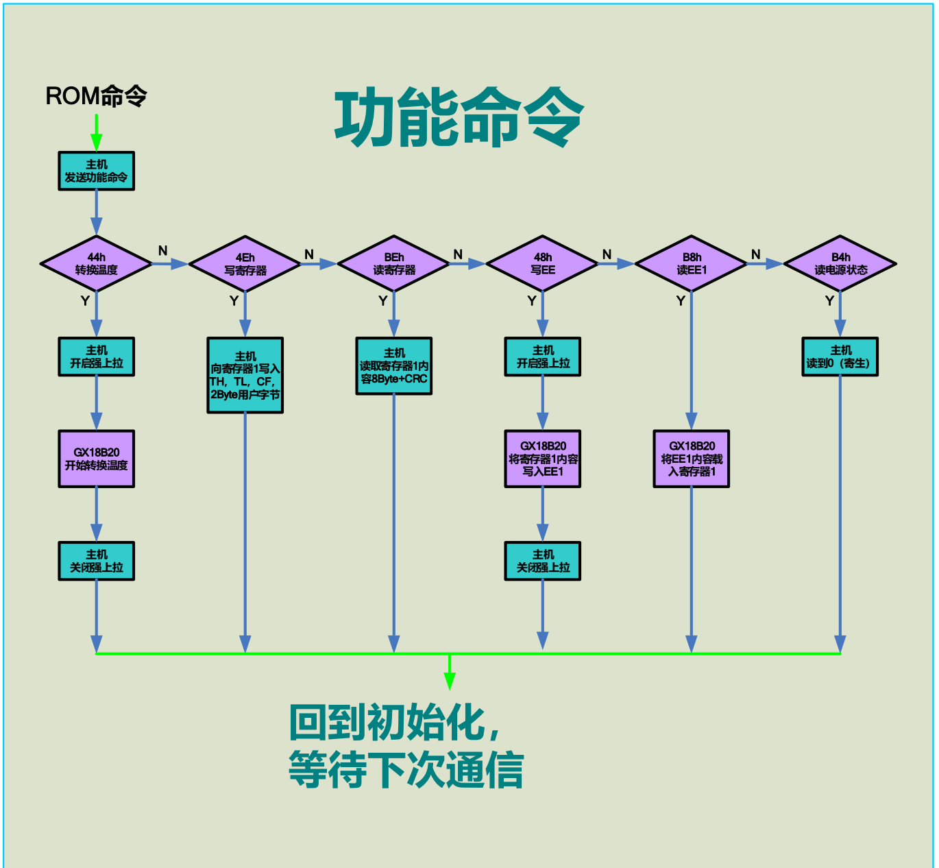
图 12. GX18B20H 功能指令流程图
