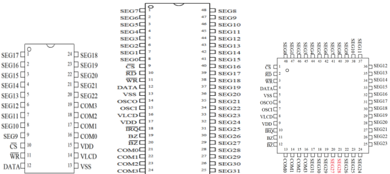
1621 SSOP24
