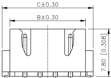
3~16 Pin样式
