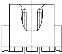
2 Pin样式
