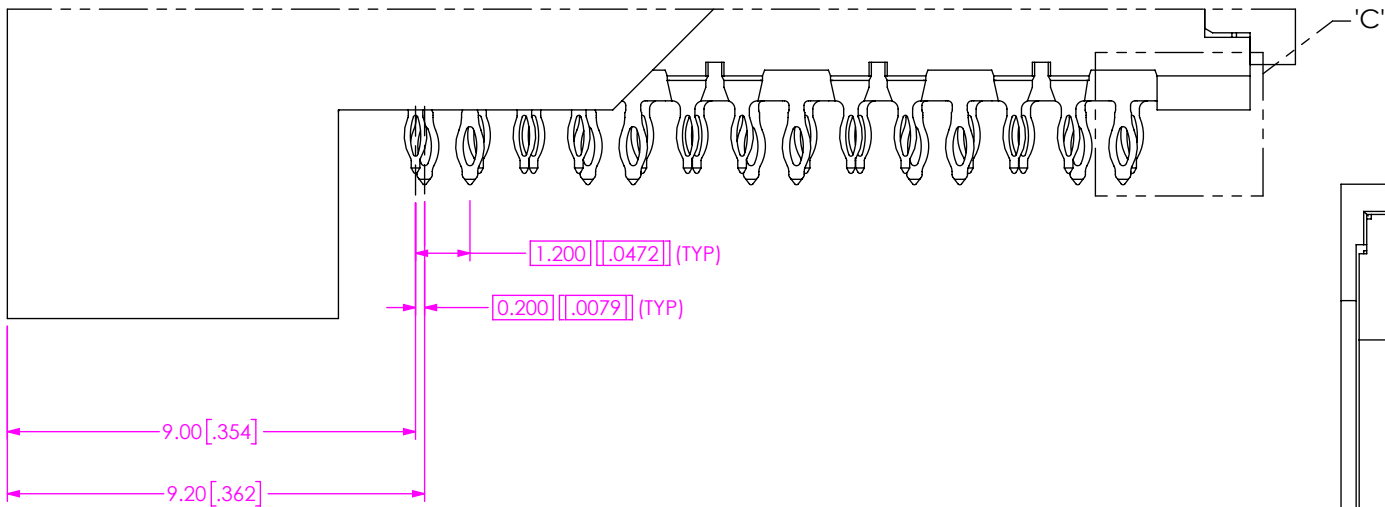
DETAIL 'B' SCALE 6 : 1
