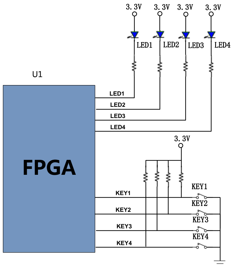
图 3-9-1 用户 LED 灯和按键硬件连接示意图
